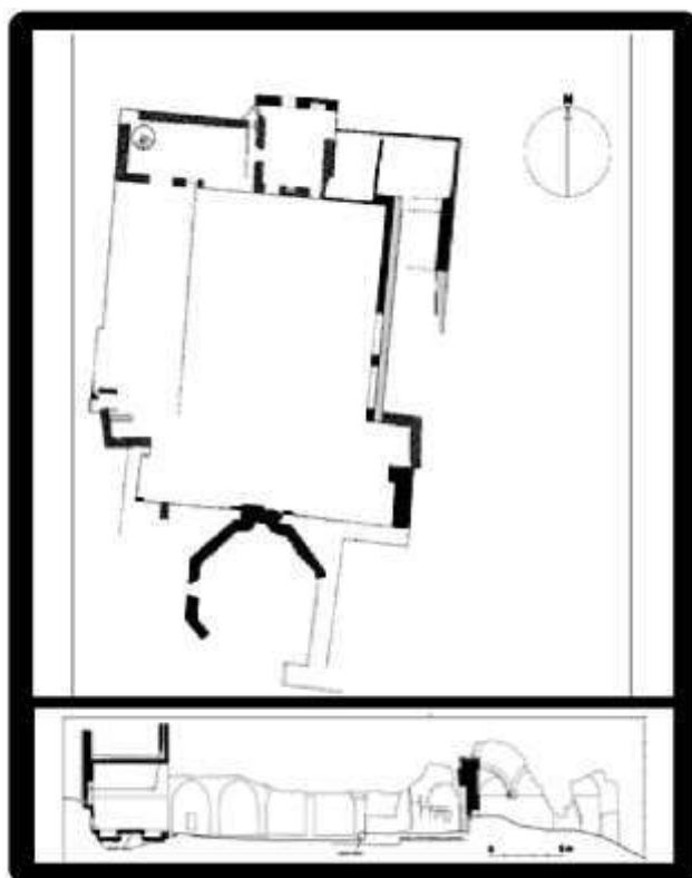
شكل (2) الطابق العلوي لمسجد ومدرسة العمادية (قبة). الباحث بعد تعديلاته عن سوبارتو
